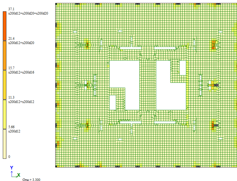
Рисунок. Требуемое верхнее армирование по X. Вторая итерация.
