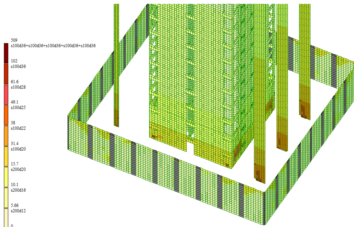
Рисунок. Требуемое горизонтальное армирование стен (максимальное по обоим сторонам). Вторая итерация.
