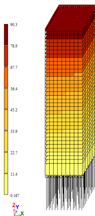
Перемещения по Y от РСН 2.3
