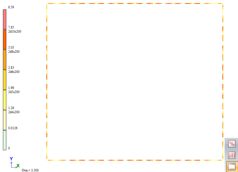
Рисунок. Требуемое поперечное армирование балок. Горизонтальное направление. Вторая итерация.
