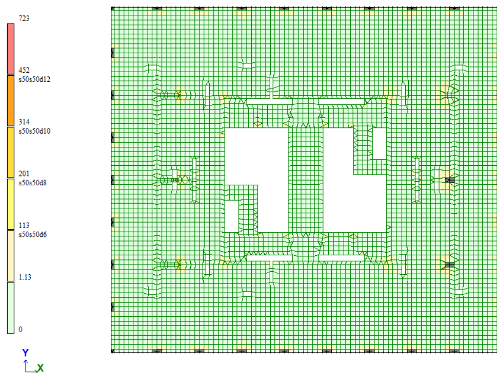
Рисунок. Требуемое поперечное армирование плит на 1м 2 . Вторая итерация.
